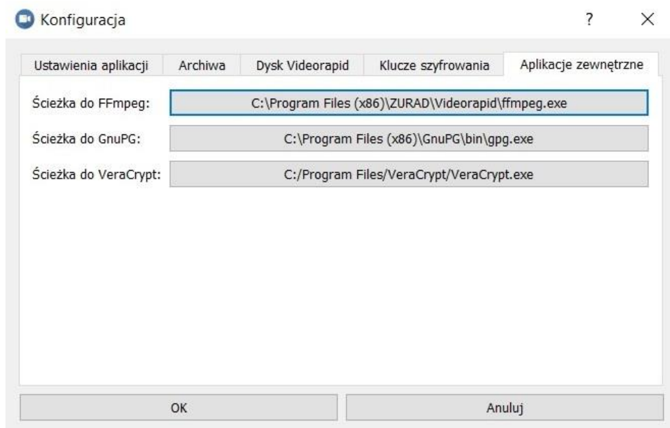
Rys. 6.5 Konfiguracja/Aplikacje zewnętrzne.
