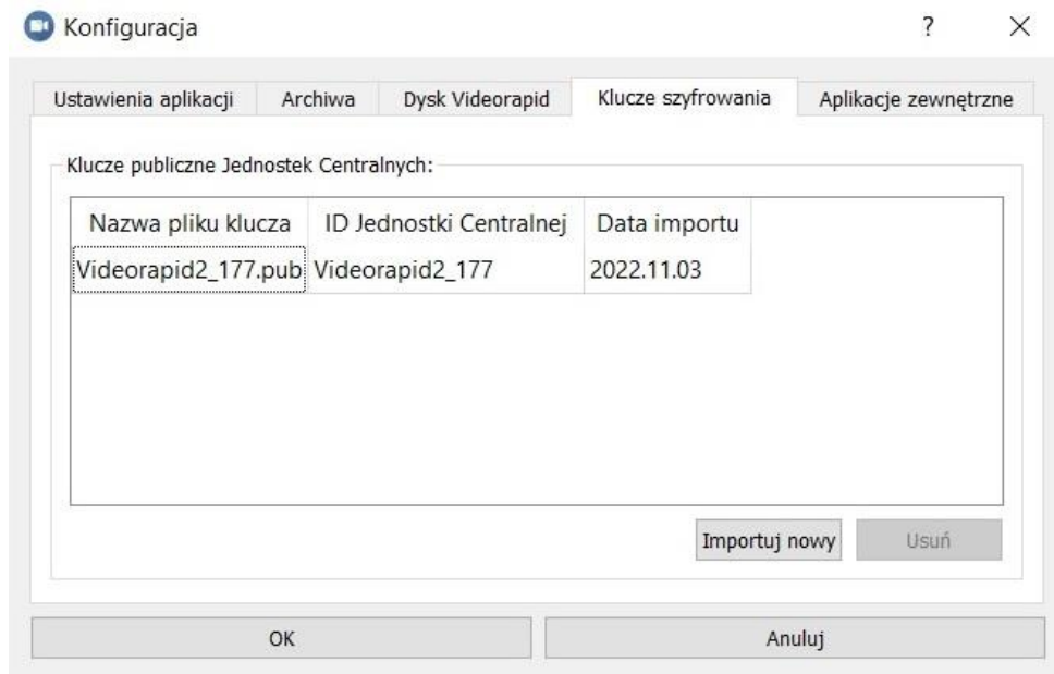
Rys. 6.4. Konfiguracja/Klucze szyfrowania.
