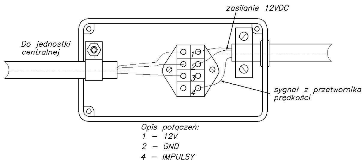
Rys. 8.1. Połączenia wewnątrz puszki połączeniowej Tacho.
