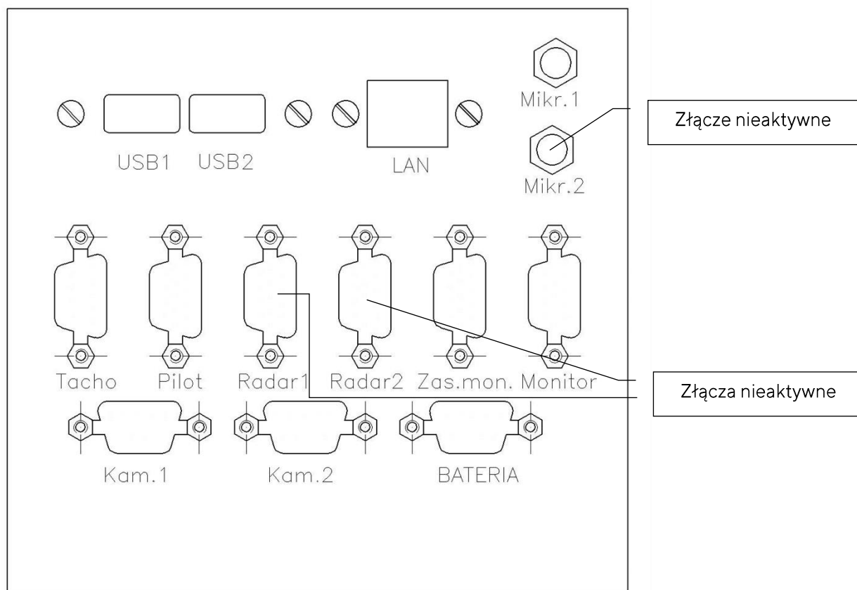
Rys. 8.2. Rozmieszczenie złączy z tyłu jednostki centralnej.
