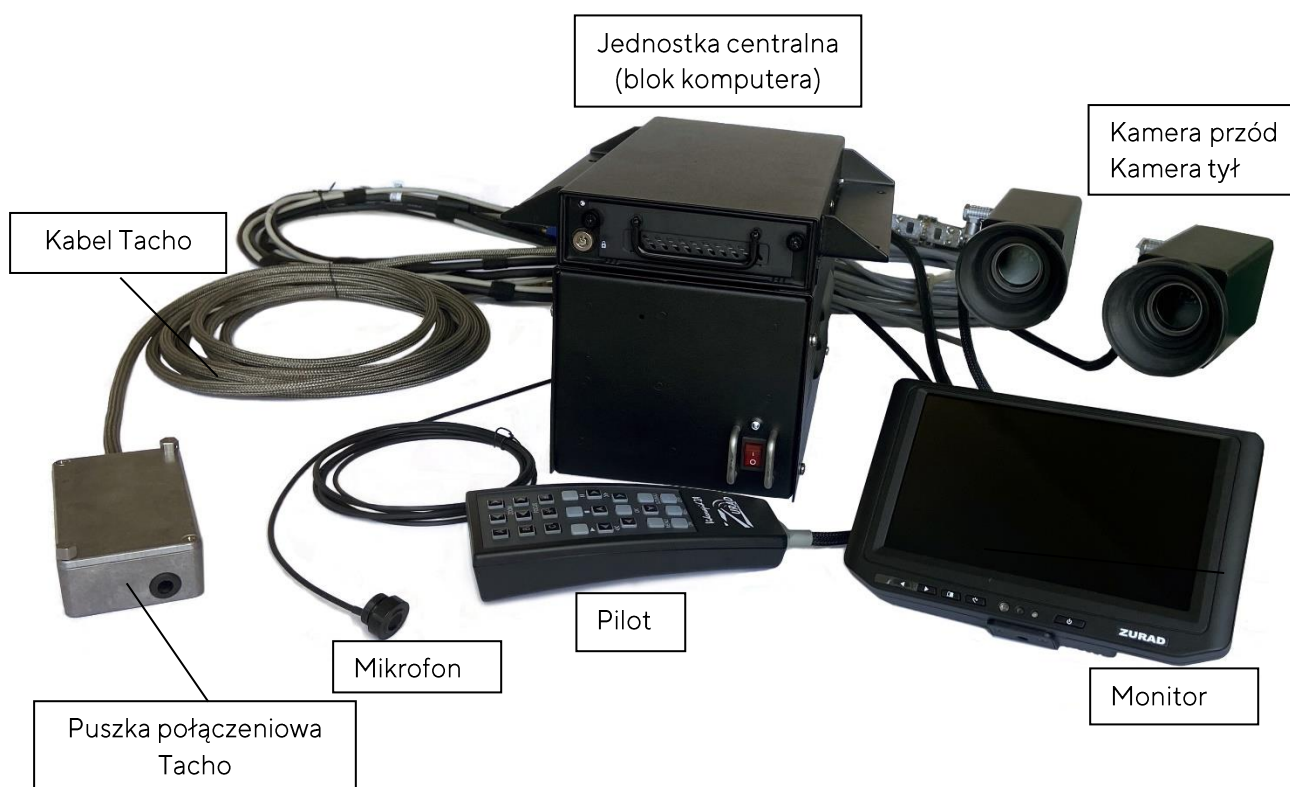
Rys. 3.1. Ukompletowanie prędkościomierza.
